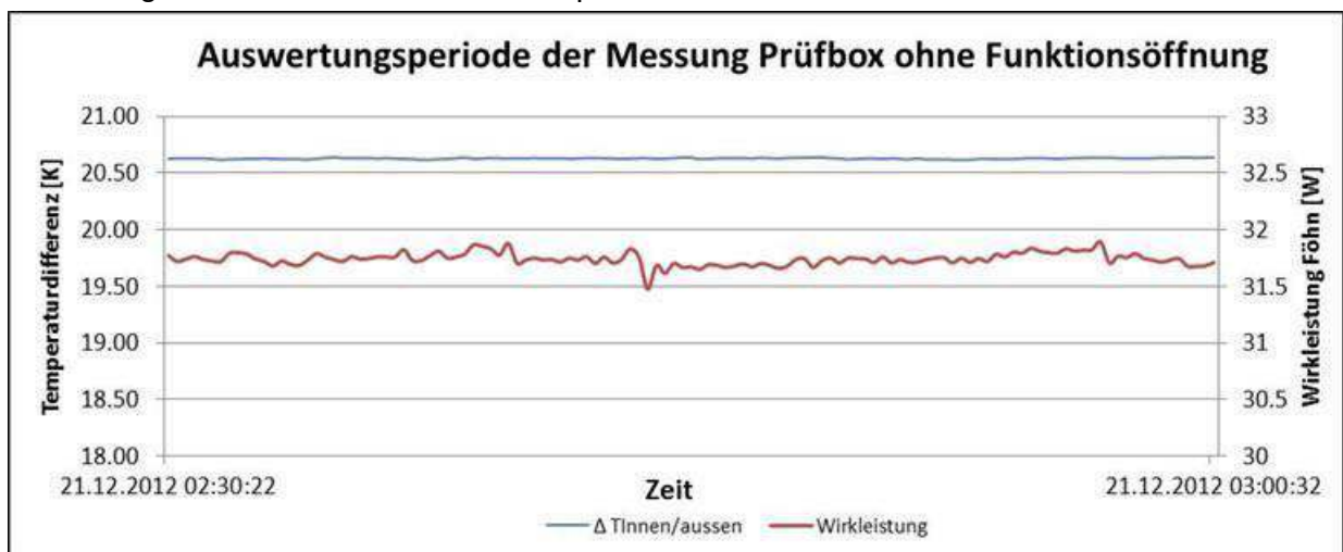
Abbildung 57: Messwerte während der Auswertungsperiode bei der Messung ohne Funktionsöffnung
