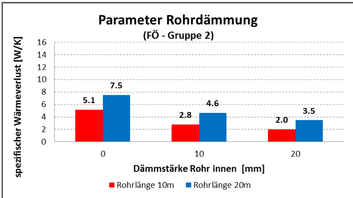
Abbildung 38: Einfluss Parameter Rohrdämmung auf den Wärmeverlust
