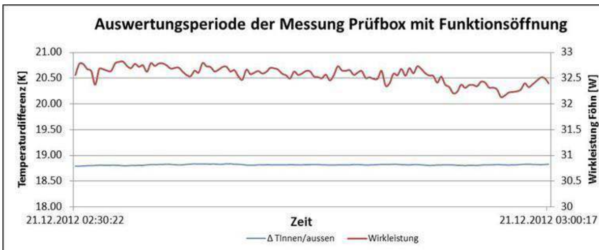
Abbildung 58: Messwerte während der Auswertungsperiode bei der Messung mit Funktionsöffnung
