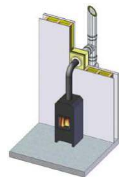
Abbildung 7: Schwedenofen mit Rauchrohr (Quelle: Edelstahlschornstein.nl)
