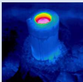
Dunstrohr - Wärmebildaufnahme
